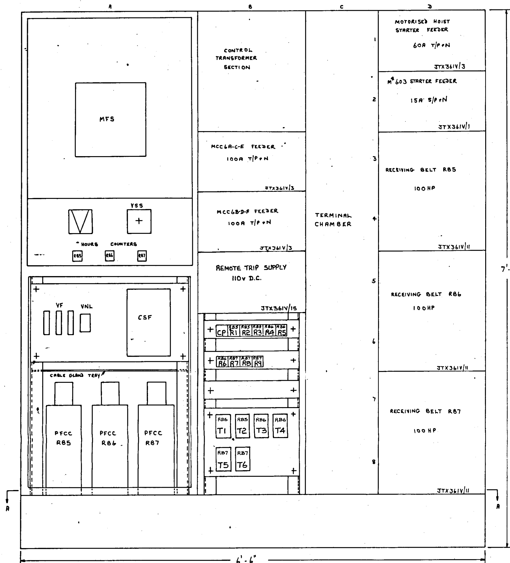
SECTION A-A
